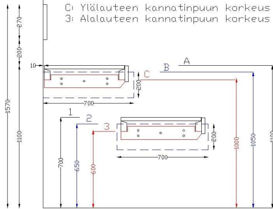
Poikkileikkauskuva. Tartuntatukien paikat korkeussuunnassa 1100 korkealla lauteella.
