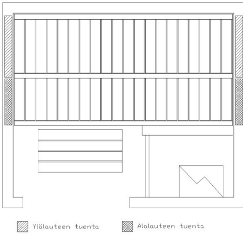
Asennuspaikat ylhäältäpäin katsottuna.
